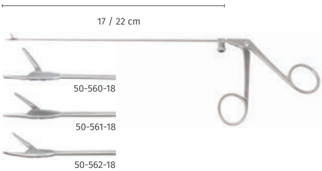
Micropinza para laringe con canal de irrigación, extrafino, cocodrilo, 1.0 mm, eje cónico (1.0 - 2.0 mm) Micro laryngeal forceps with irrigation channel, very fine, alligator jaws, 1.0 mm, conical shaft (1.0 - 2.0 mm)
