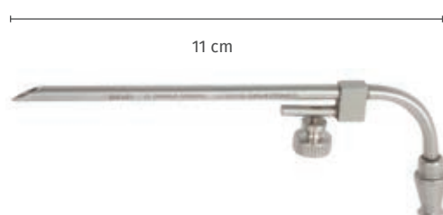
Cánula Timer para inyección para laringoscopios rígidos y extensibles tamaños 1 hasta 7, 11 cm
