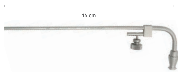
Tubo para evacuación de humo, para laringoscopios rígidos y extensibles tamaños 3 hasta 7, 14 cm
