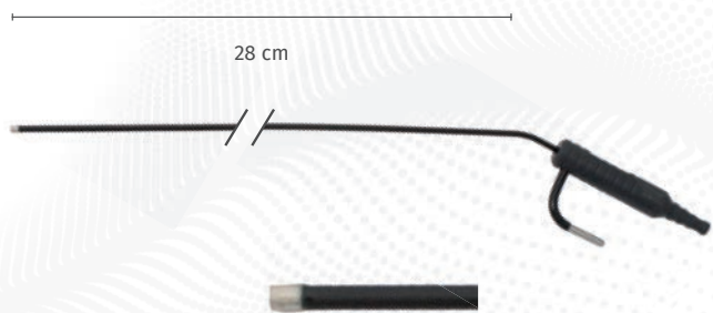
Tubo de aspiración coagulador monopolar, NON-STICK, angulado, DE 4 mm, esfera 4 mm, longitud de trabajo 28 cm Coagulation suction tube, monopolar, NON-STICK, angled, 4 mm OD, 4 mm ball end, suction control, 28 cm working length
